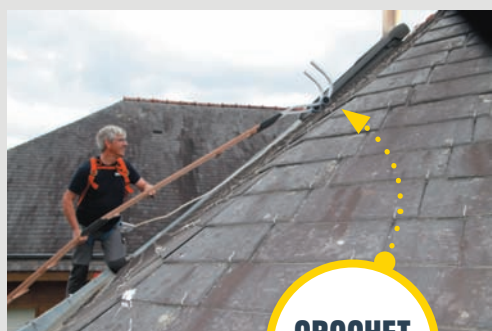
CROCHET ALU
