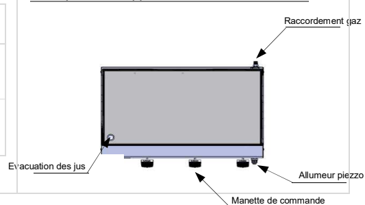
Description de l'appareil Plancha en vue dessus
